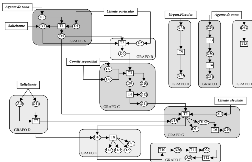
Fig. 5. Factorización de los Grafos BUC para los procesos de la organización
