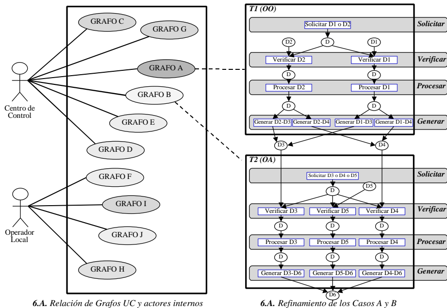
Fig. 6. Relación de los Grafos UC con los actores y refinamiento de los grafos de casos A y B.
