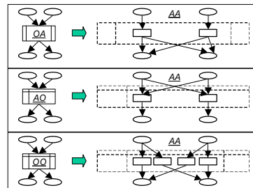
2.D. Estandarización de las tareas OA, AO y OO de los GCM.
