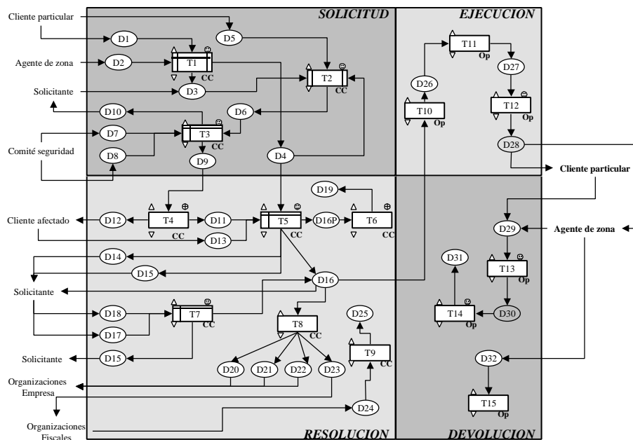
Fig. 3. Grafo de Casos para cuatro procesos en dos secciones de una organización
