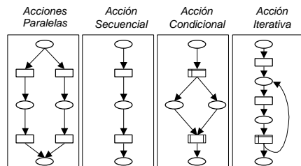
2.C. Los cuatro tipos de flujo de acción básicos para el modelado de casos de uso con GCM
