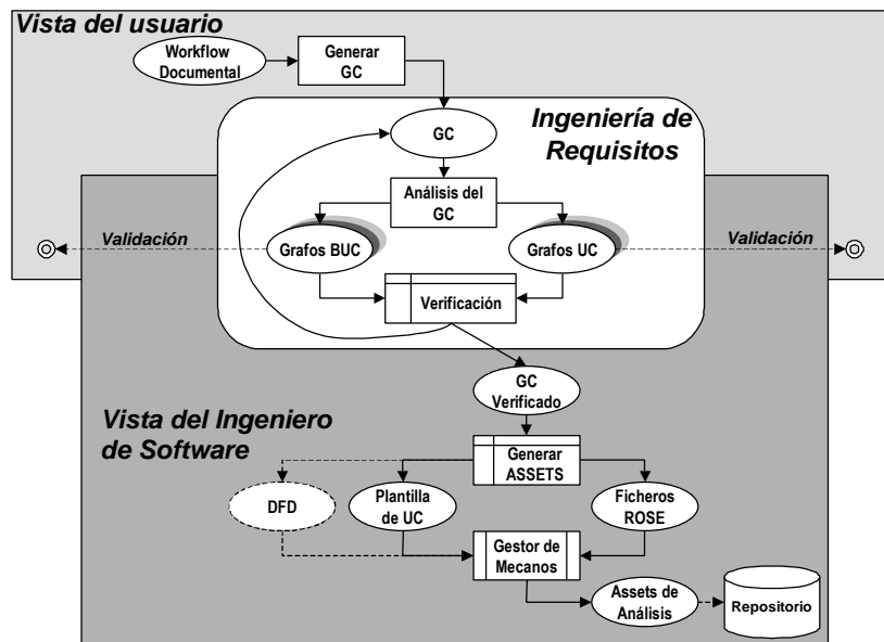
Fig. 1. Marco general de trabajo para la normalización de la captura de los requisitos de usuario.
