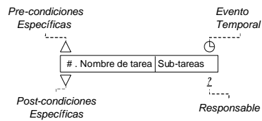
2.B. Representación gráfica de una tarea genérica en un GC
